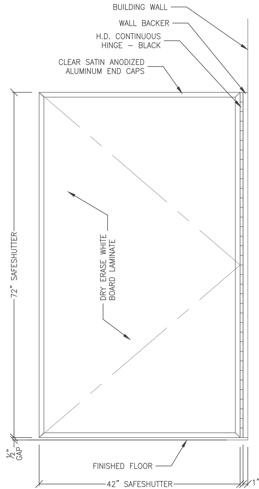
1 ELEVATION 2.5 SCALE: 1" = 1'-0"
