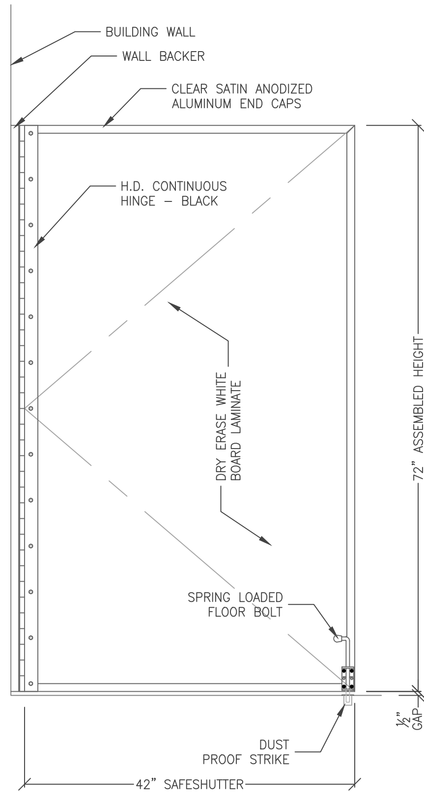
3 ELEVATION 2.5 SCALE: 1" = 1'-0"
