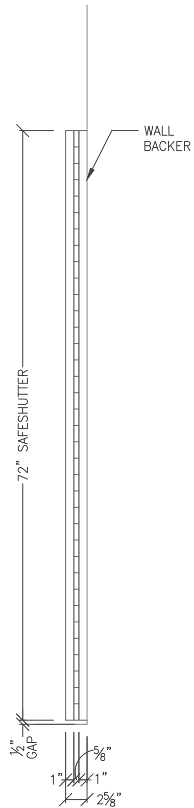
2 ELEVATION 2.5 SCALE: 1" = 1'-0"
