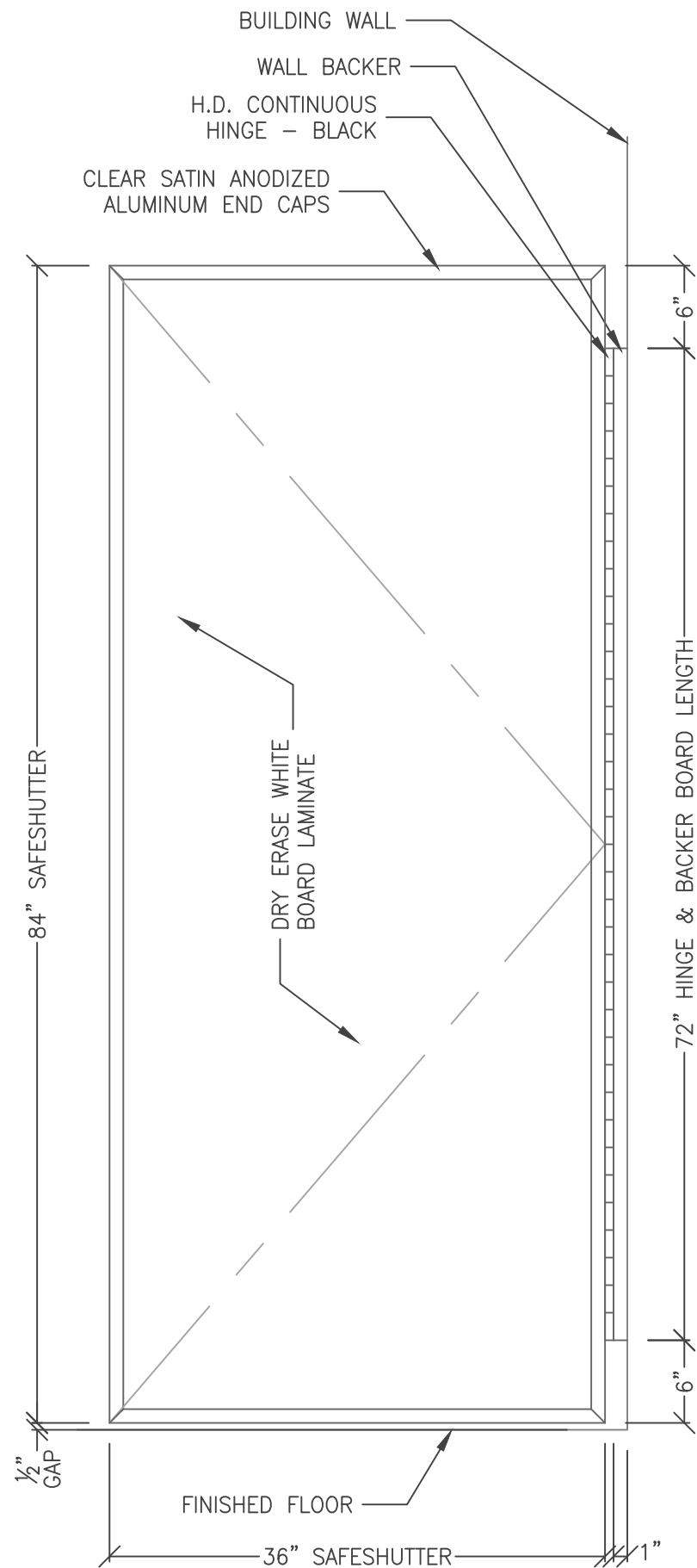
1 ELEVATION 2.3 SCALE: 1" = 1'-0"
