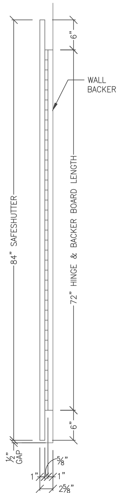
2 ELEVATION 2.3 SCALE: 1" = 1'-0"
