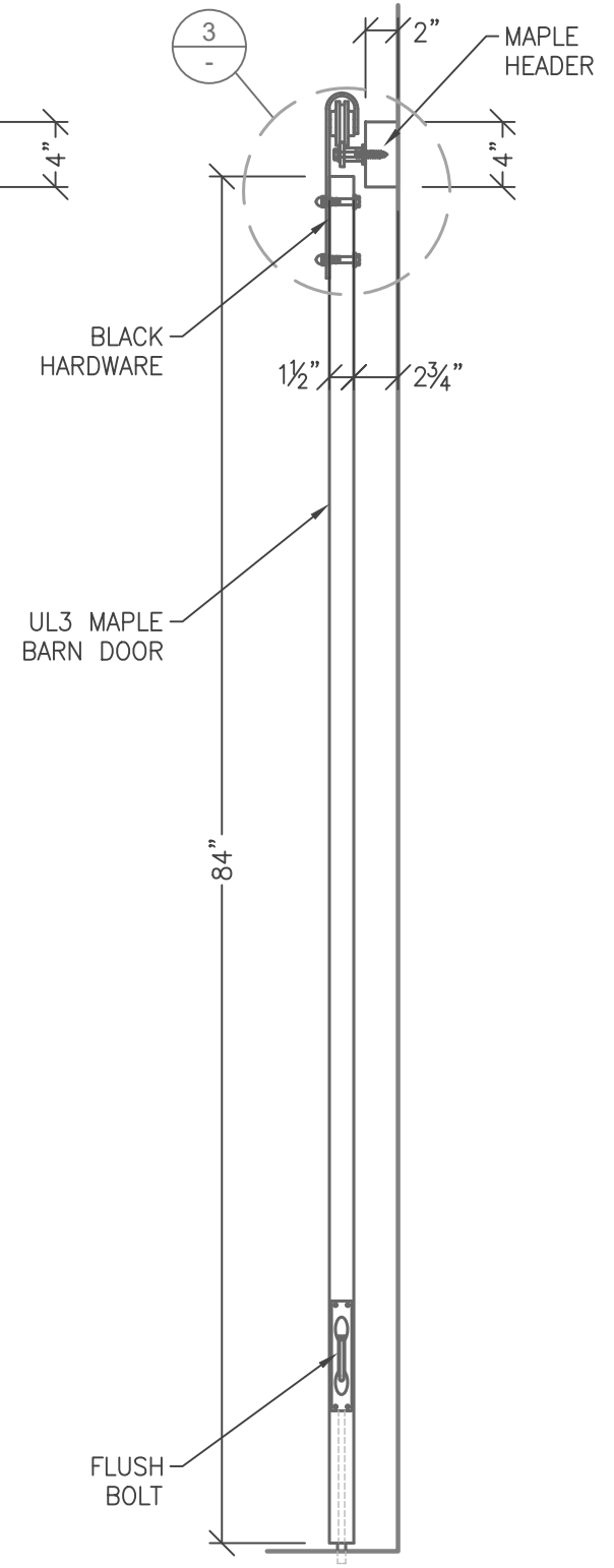
2 SIDE VIEW 3.13 SCALE: 1" = 1'-0"
