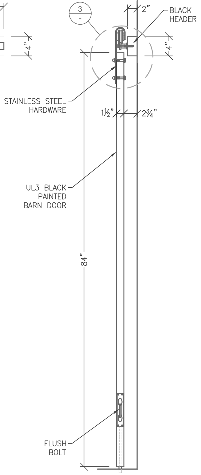
2 SIDE VIEW 3.63 SCALE: 1" = 1'-0"
