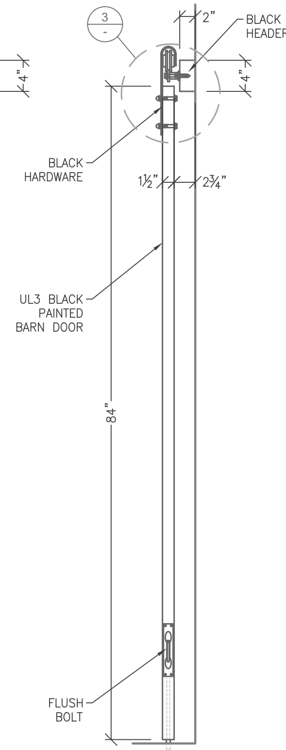
2 SIDE VIEW 3.73 SCALE: 1" = 1'-0"
