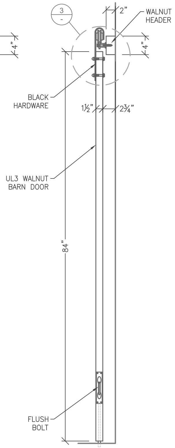
2 3.32 SIDE VIEW SCALE: 1" = 1'-0"
