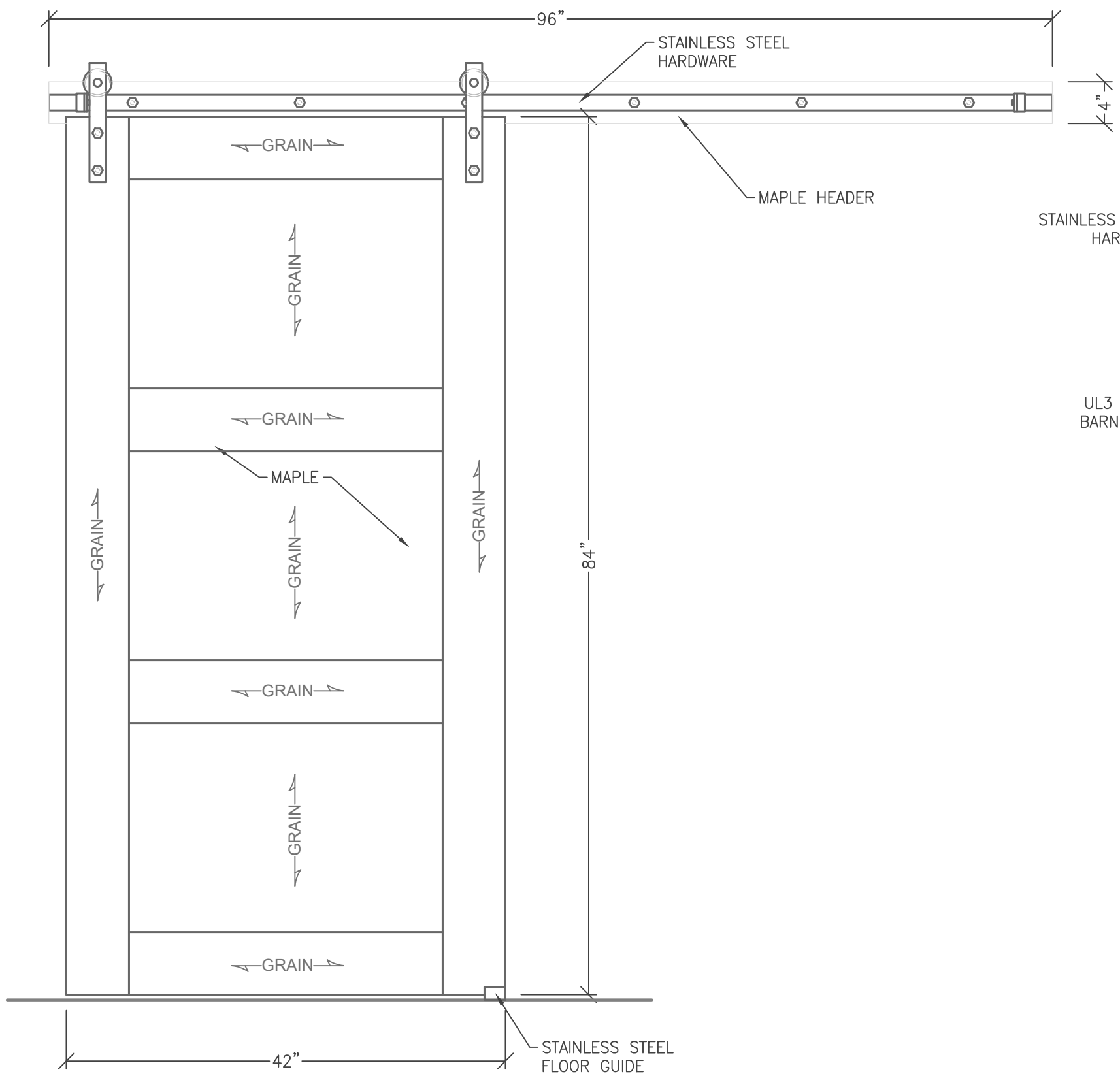
1 3.1 UL3 B.R. BARN DOOR BD-3P-3670-MAPSS-UL03 SCALE: 1" = 1'-0"
