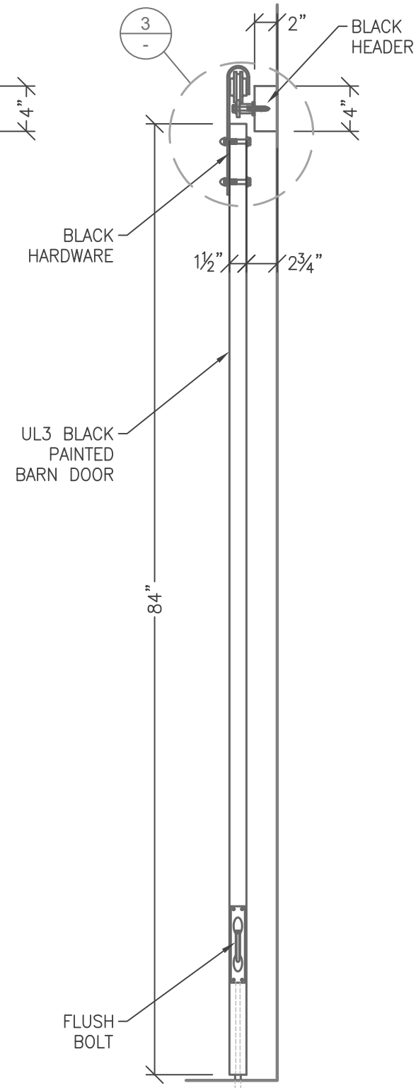
2 SIDE VIEW 3.71 SCALE: 1" = 1'-0"
