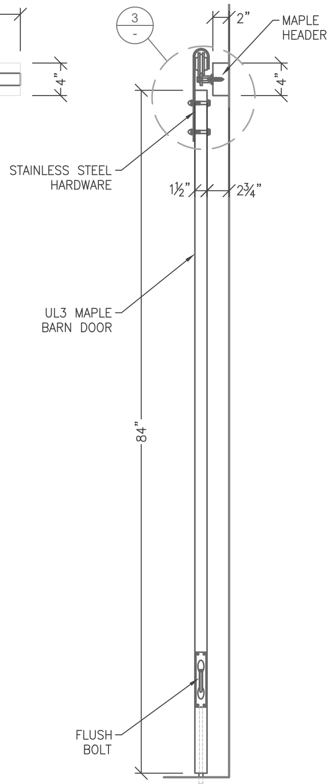
2 3.0 SIDE VIEW SCALE: 1" = 1'-0"
